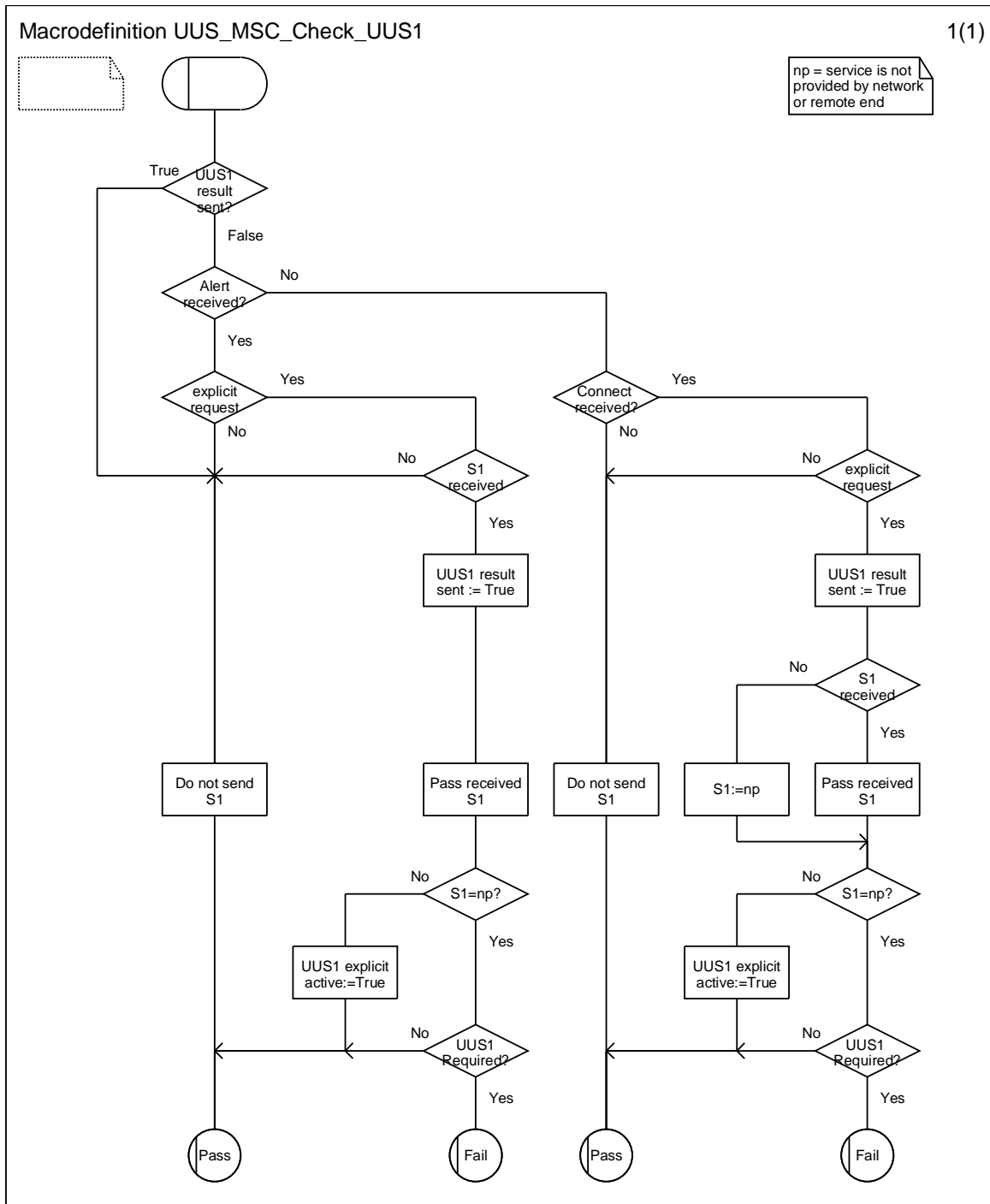
Figure 9.3.7: Macrodefinition UUS_MSC_Check_UUS1
