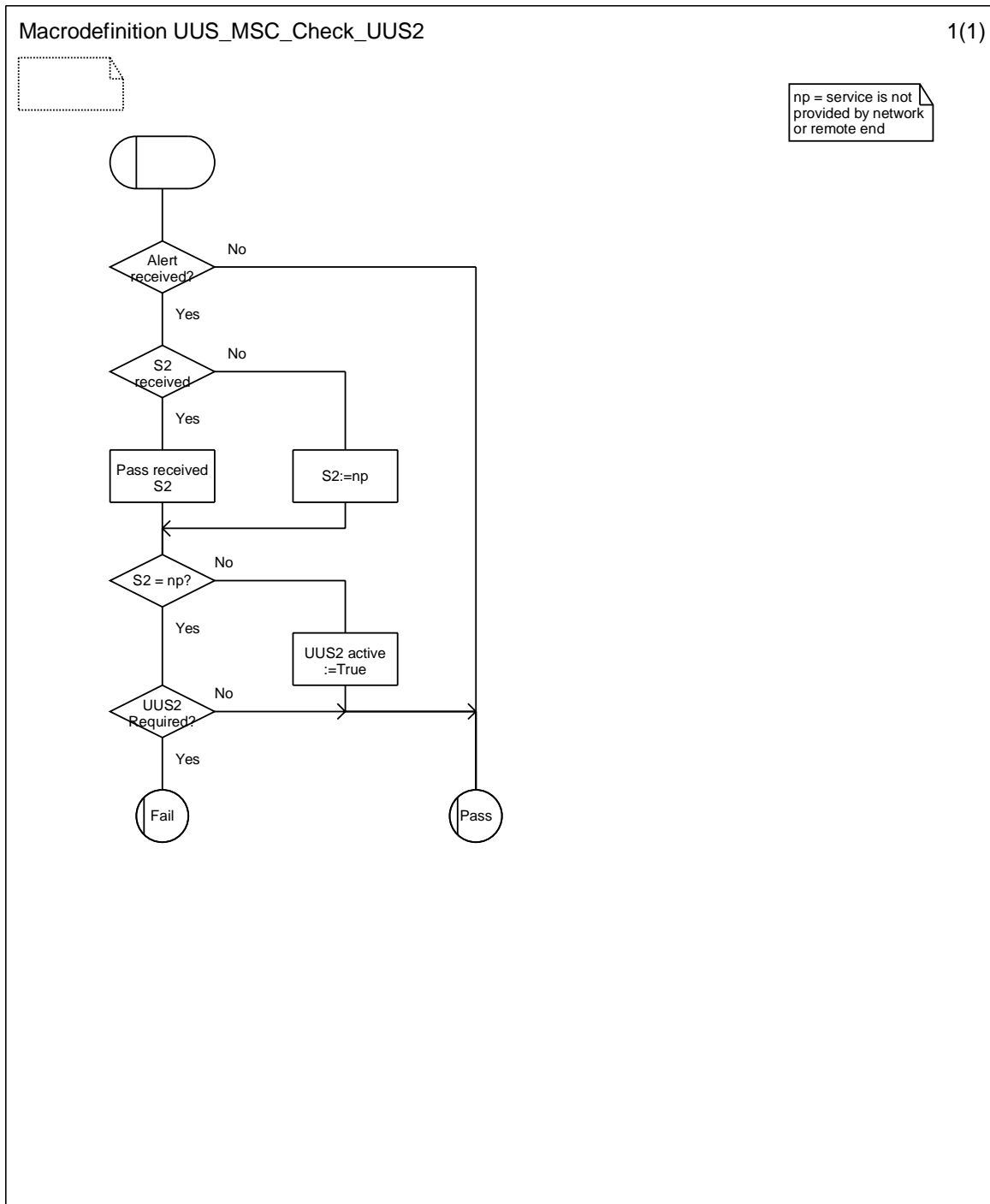
Figure 9.3.8: Macrodefinition UUS_MSC_Check_UUS2
