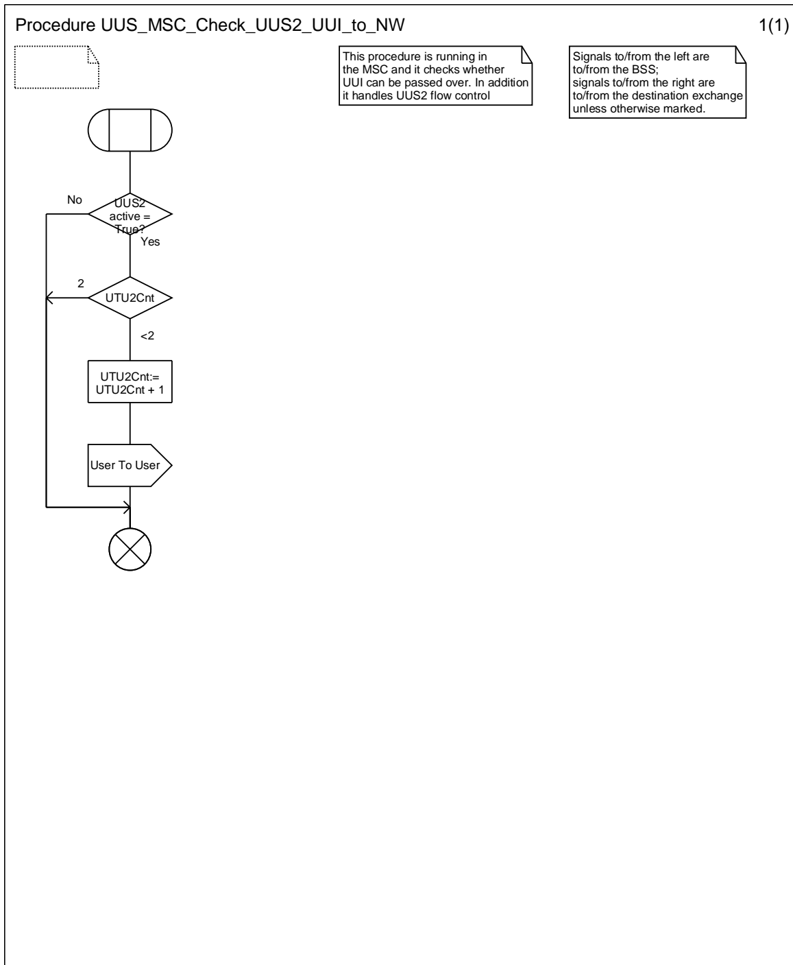
Figure 9.3.3: Procedure UUS_MSC_Check_UUS2_UUI_to_NW
