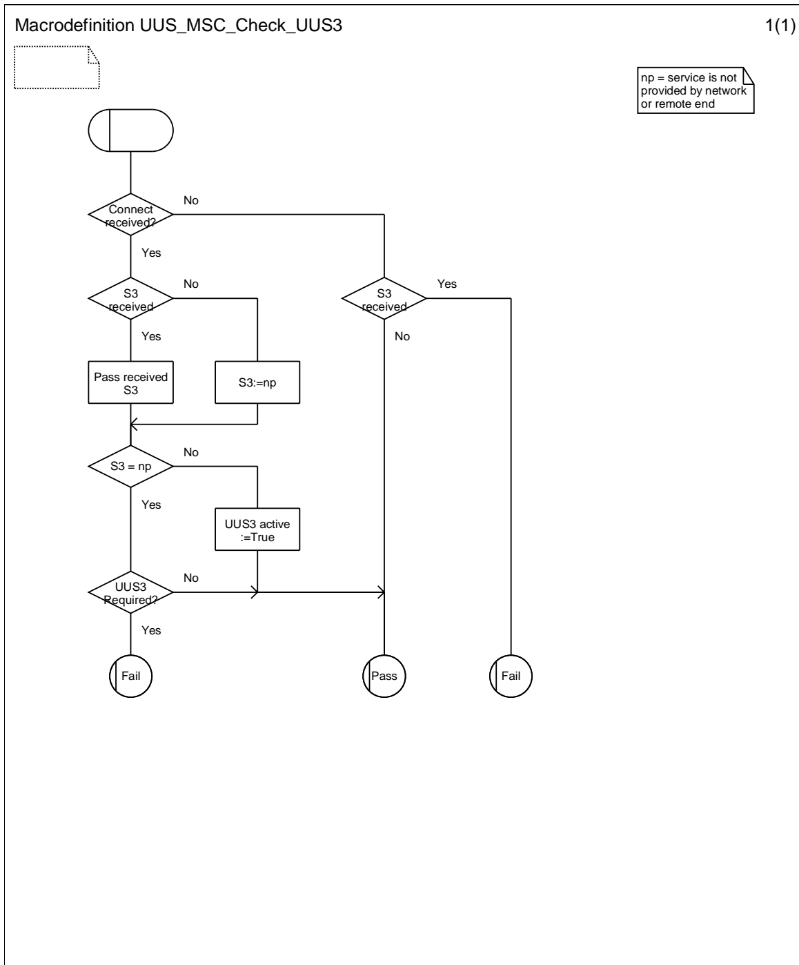
Figure 9.3.9: Macrodefinition UUS_MSC_Check_UUS3
