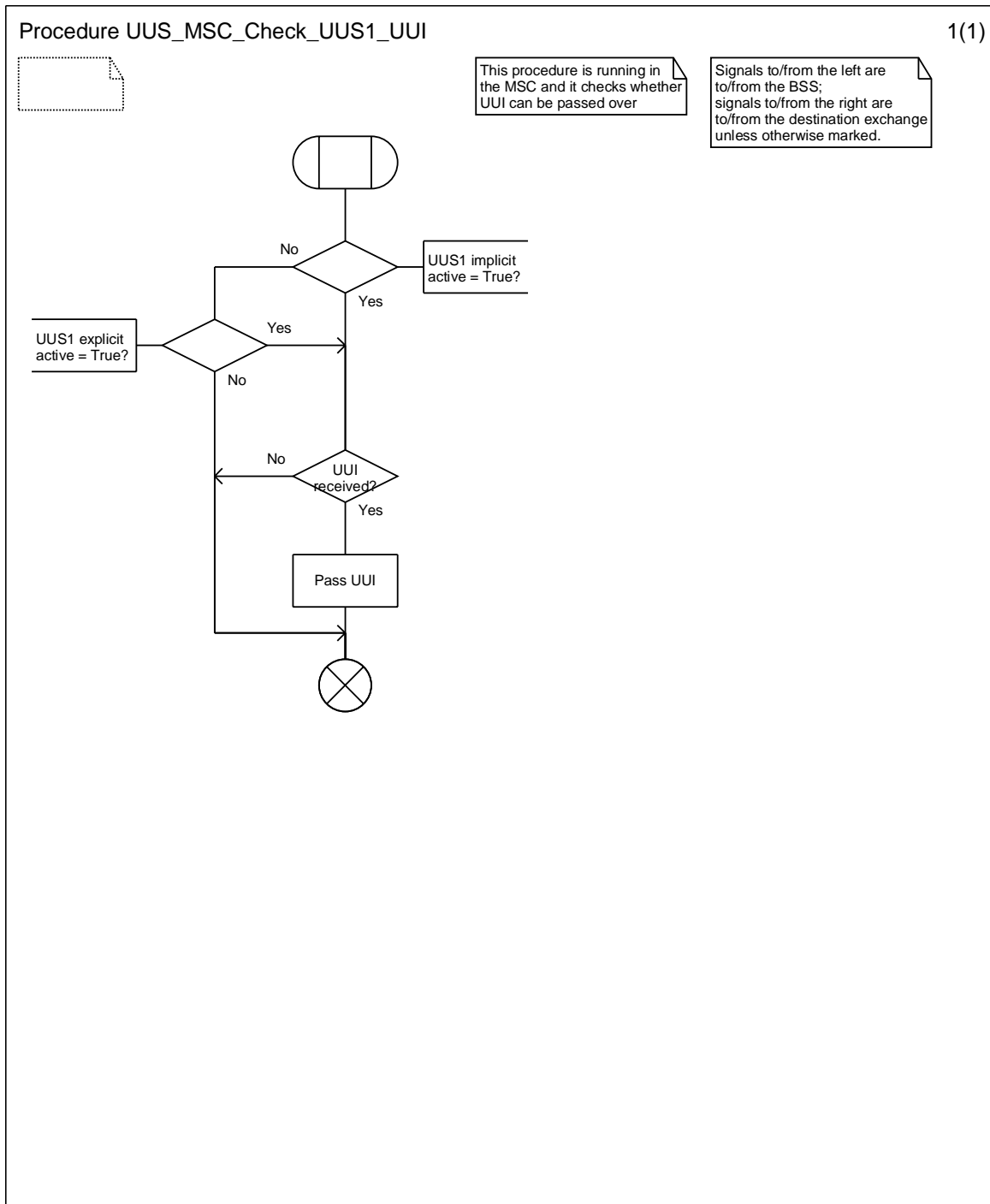
Figure 9.3.1: Procedure UUS_MSC_Check_UUS1_UUI
