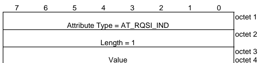
Figure 8.1.1.1-1: AT_RQSI_IND attribute
