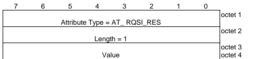
Figure 8.1.1.2-1: AT_RQSI_RES attribute.
