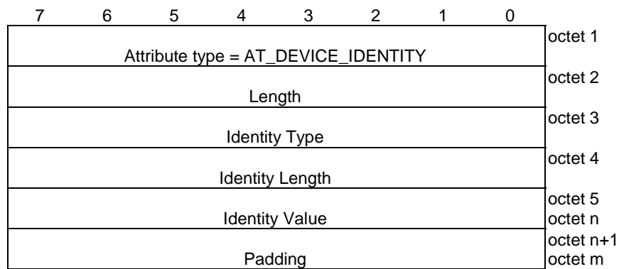
Figure 8.2.8.1-1: AT_DEVICE_IDENTITY attribute
