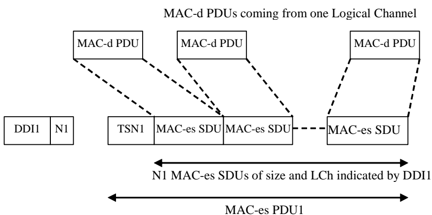
Figure 9.1.5.1 MAC-es PDU
