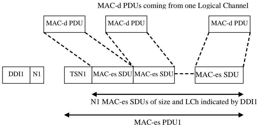
Figure 9.1.5.1 MAC-es PDU
