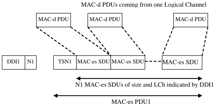
Figure 9.1.5.1 MAC-es PDU
