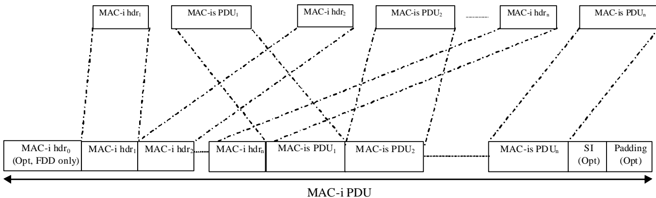
Figure 9.1.5.4a: MAC-i PDU.
