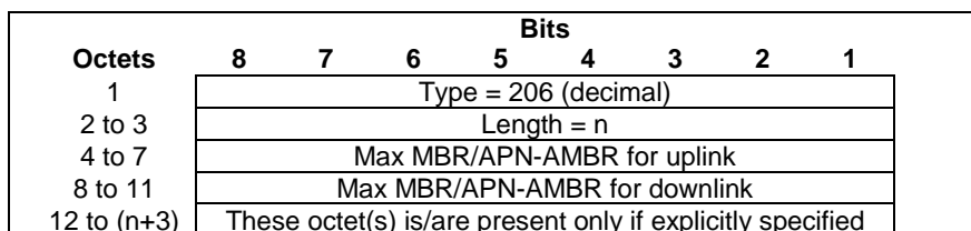
Figure 7.7.106-1: Max MBR/APN-AMBR
